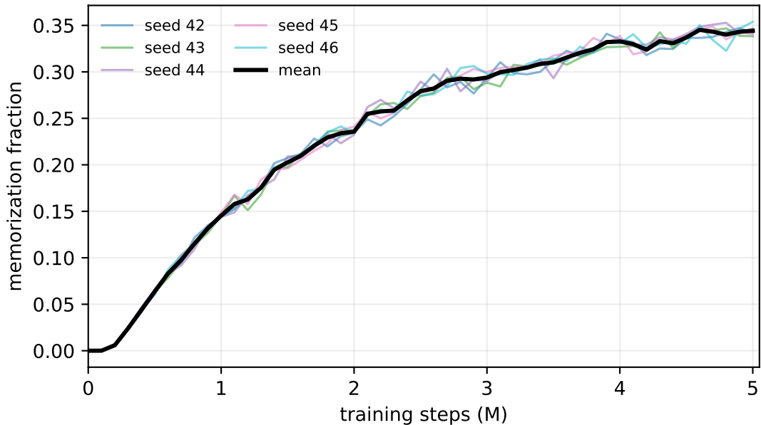
CelebA d=30
